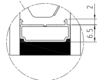
CANALINA RIBASSATA CON INCASTRO
