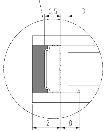
CANALINA RIBASSATA CON ALETTA
